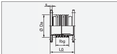
Typ AFN mit Leitrohr
