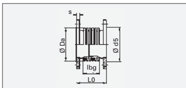
Typ ABN mit Leitrohr
