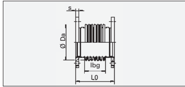
Typ AFN ohne Leitrohr
