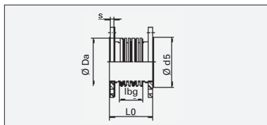
Typ ABN ohne Leitrohr
